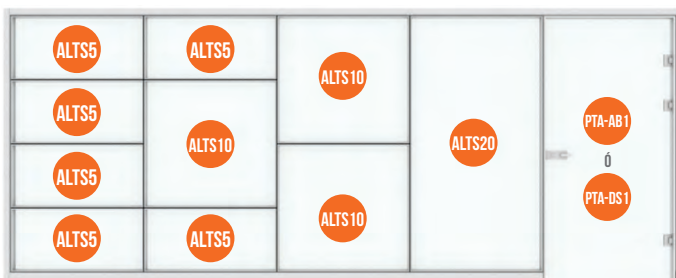
ALTURA DE 2170 MM, PANEL SENCILLO
