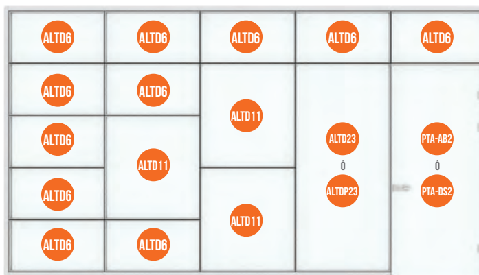
ALTURA DE 3019 MM, PANEL DOBLE
